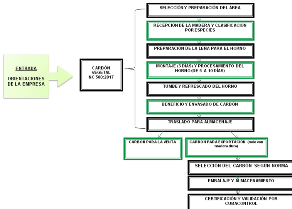
Figura: 2 Flujo diagrama de la Producción de Carbón Vegetal.
